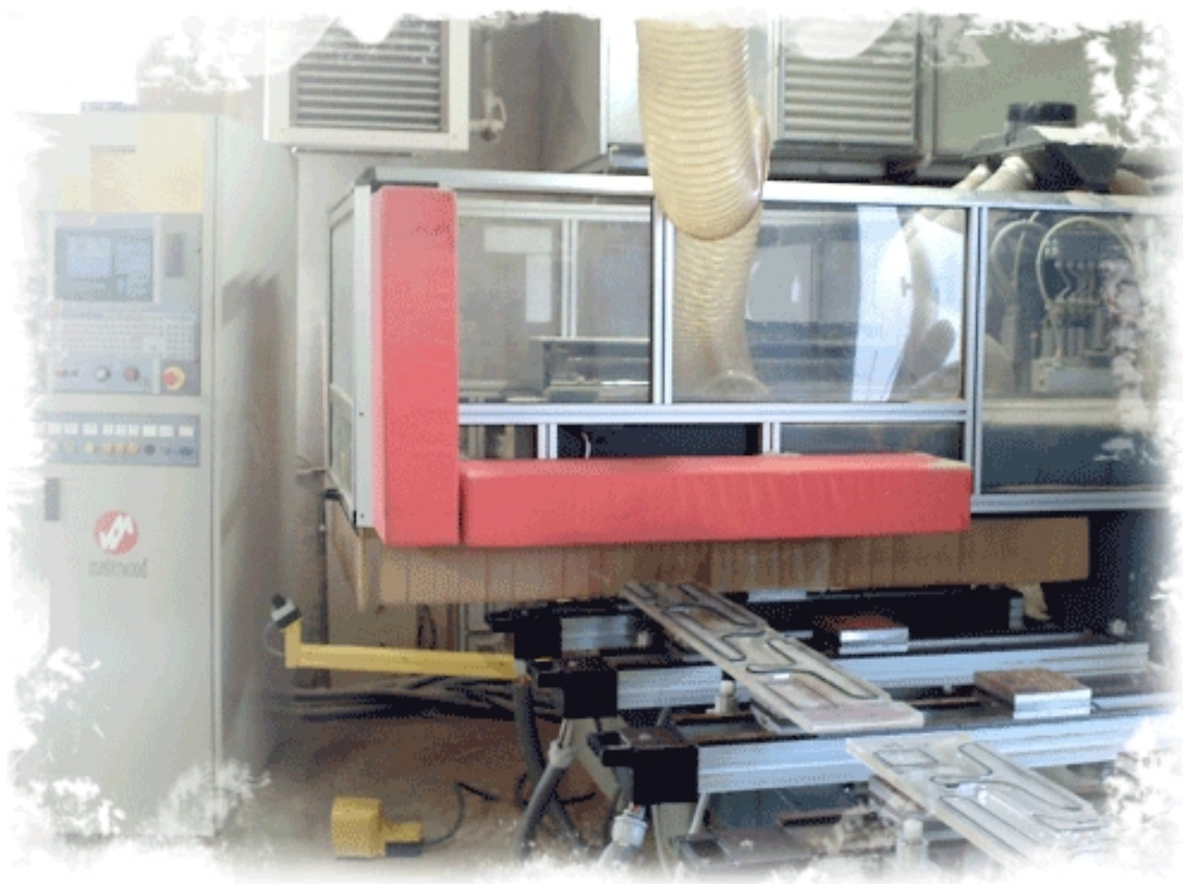
Machine à commande numérique
